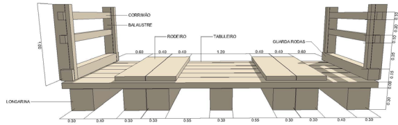
1 Detalhe 3D Escala 1/50
