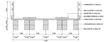
C Corte 01 Escala 1/50
